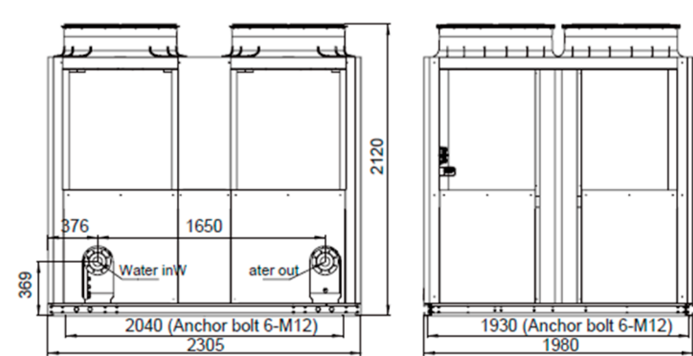
LSQWF130VM/NaA-M (Unit:mm)
