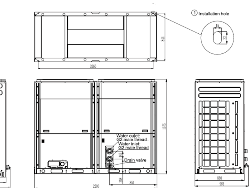
LSQWF65VM/NaA-M (Unit:mm)
