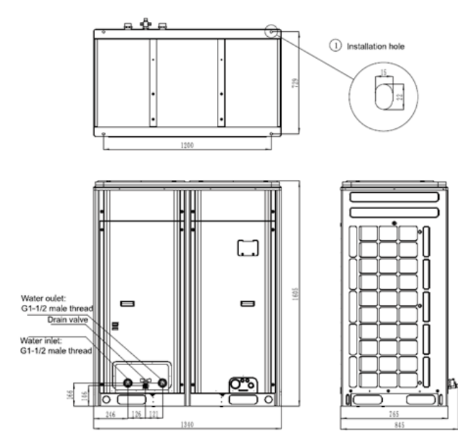
LSQWF35VM/NaA-M (Unit:mm)
